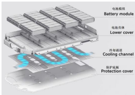
图 1：动力电池结构件示意图
