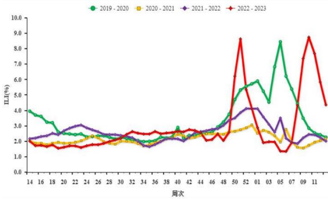
图表1: 北方省份哨点医院: 流感样病例百分比 (至 2023 第 13 周)
