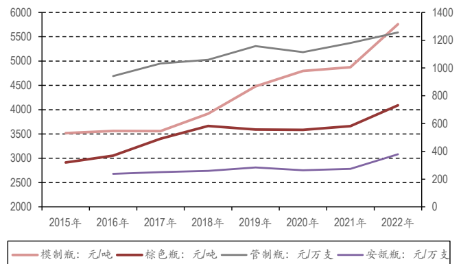
图表 4. 产品单价均有上升趋势，模制瓶价格涨幅较大
