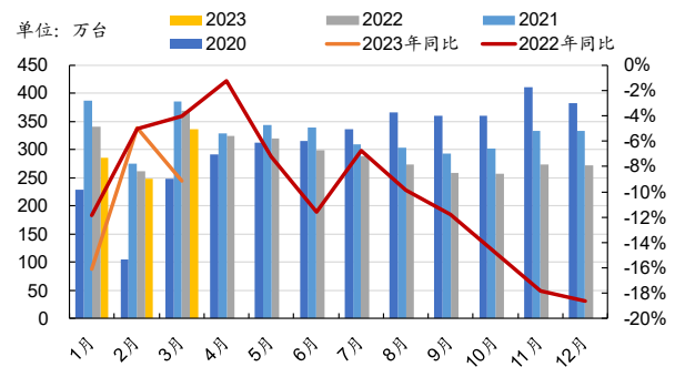
图 28: 冰柜销量
