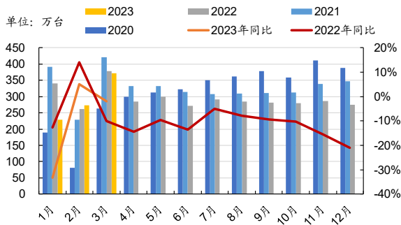
图 27: 冰柜产量
