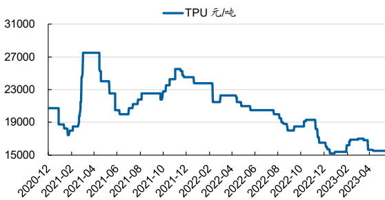
图 71: TPU 价格
