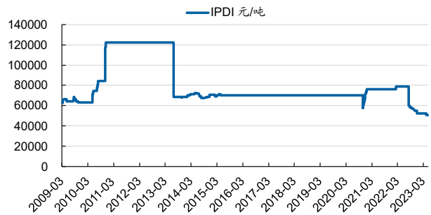
图 66：IPDI 市场价
