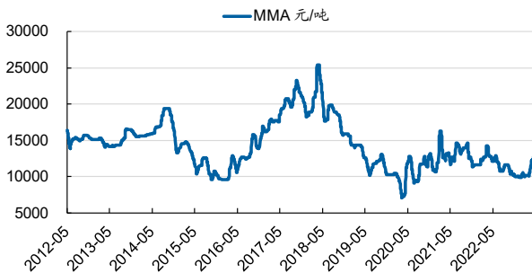
图 69: MMA 市场价
