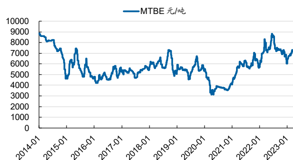
图 63: MTBE 价格
