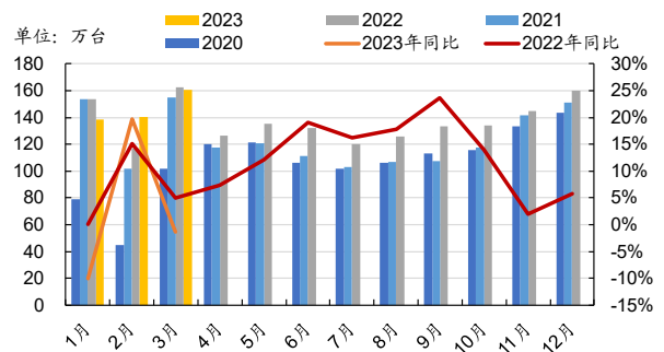
图 30: 冰柜内销量
