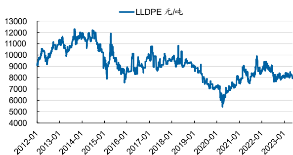
图 58: LLDPE 价格
