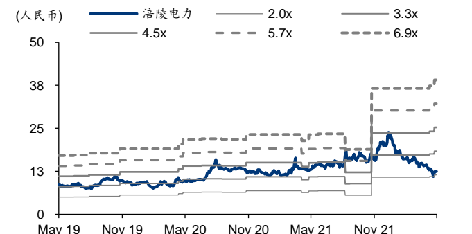
图表7: 涪陵电力 PB-Bands
