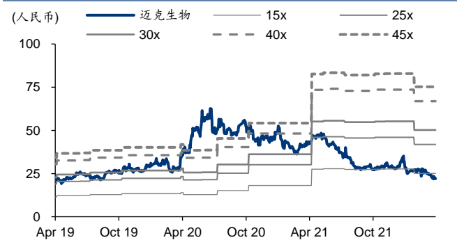
图表4: 迈克生物 PE-Bands
