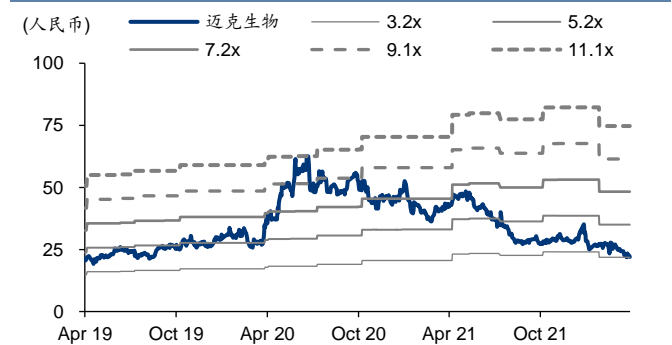
图表5: 迈克生物 PB-Bands
