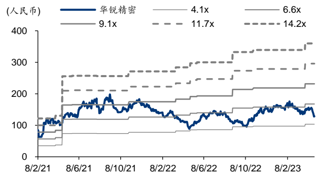
图表3: 华锐精密 PB-Bands
