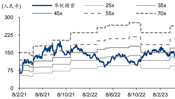
图表2: 华锐精密 PE-Bands
