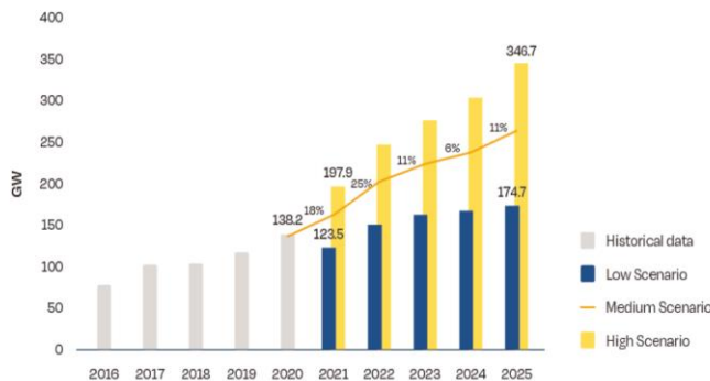
图21：2025 年全球光伏市场的新增装机容量将达到 266GW
