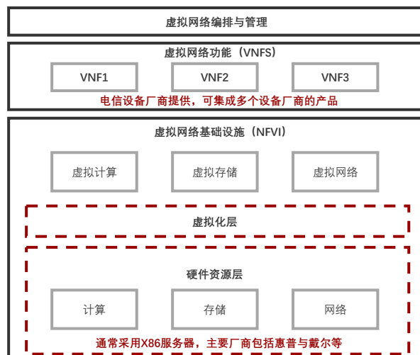
NFV架构
