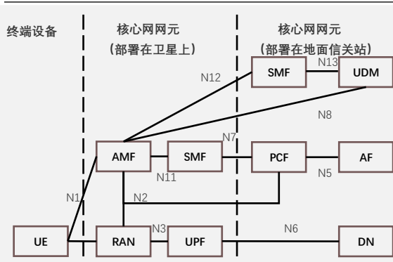
卫星核心网与5G融合拓扑图
