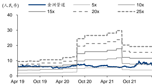
图表3: 金洲管道 PE-Bands
