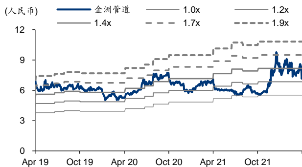
图表4: 金洲管道 PB-Bands
